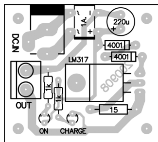
การลงอุปกรณ์วงจรประจุแบตเตอรี่
