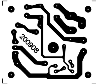
สายทองแดงวงจรประจุแบตเตอรี่
